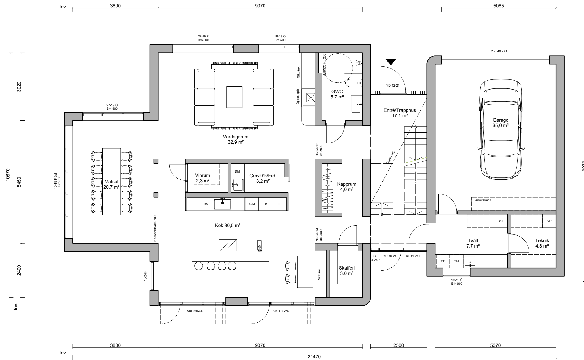
Plan 1 - Entréplan 1:100 (A3)
